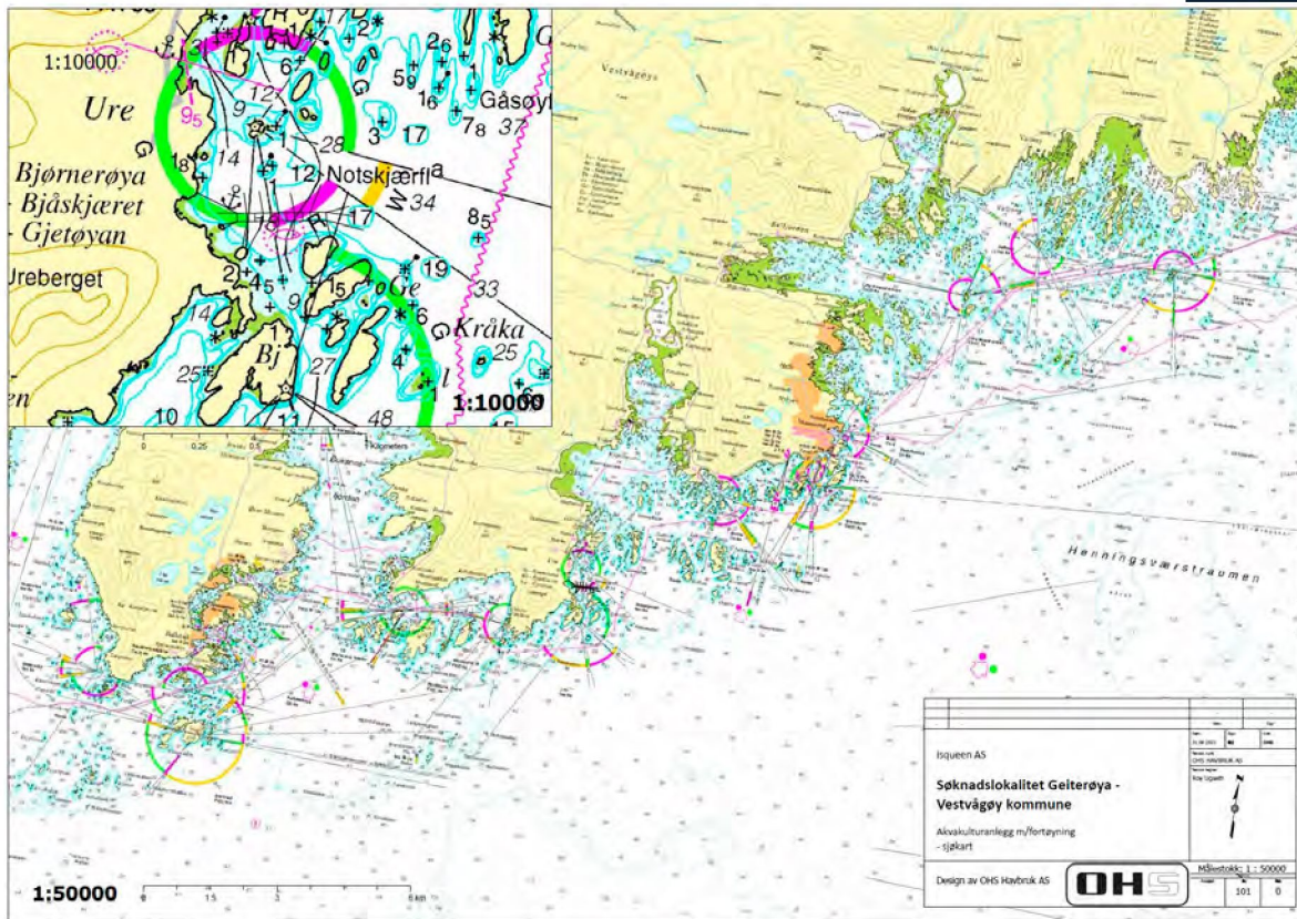
Figur 2: Utsnitt av sjøkart som viser anleggets plassering og lyktesektorer.
